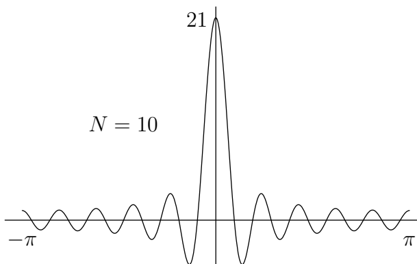
Σχήμα 8: Ο πυρήνας του Dirichlet
