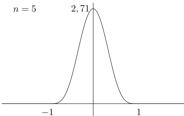
Σχήμα 3: Η συνάρτηση K_n(x) για n = 5 .
