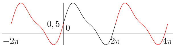
Σχήμα 5: Η διαδικασία της επέκτασης μιας συνάρτησης σε περιοδική (περιοδικοποίηση). Το γράφημα στα διαστήματα [-2\pi, 0] και [2\pi, 4\pi] είναι μεταφορές του γραφήματος στο διάστημα [0, 2\pi]
