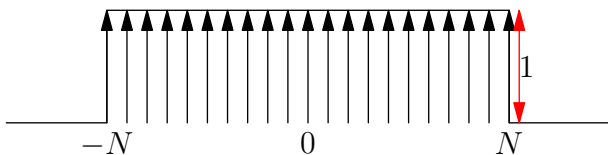
Σχήμα 9: Οι συντελεστές Fourier του πυρήνα του Dirichlet D_N(x) για N = 10
