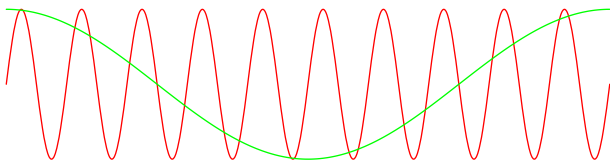
Σχήμα 4: Μια συνάρτηση που είναι «πιο συνεχής» από μια άλλη
