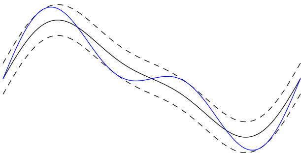
Σχήμα 6: Η βέλτιστη πολυωνυμική προσέγγιση (μπλε) της συνάρτησης πρέπει να ακουμπάει και το σύνορο της \rho -ζώνης (διακεκομμένη γραμμή) και προς τα πάνω και προς τα κάτω. Εδώ \rho = \|f - p^*\|_\infty .
